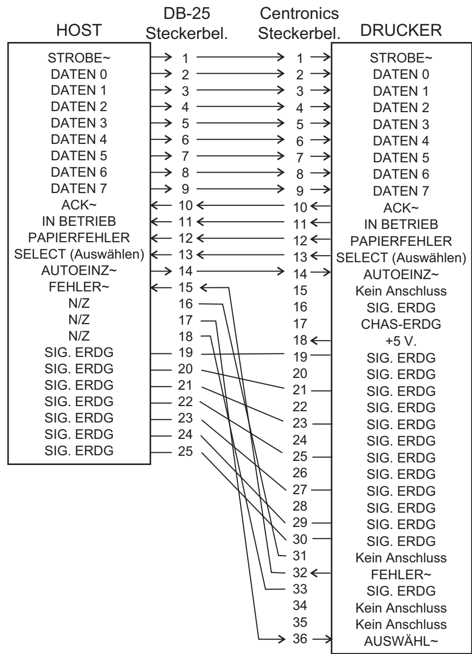
DB-25 zu Centronics (Kabel)
